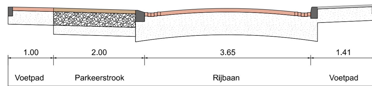
Dwarsprofiel A-A 1:50
