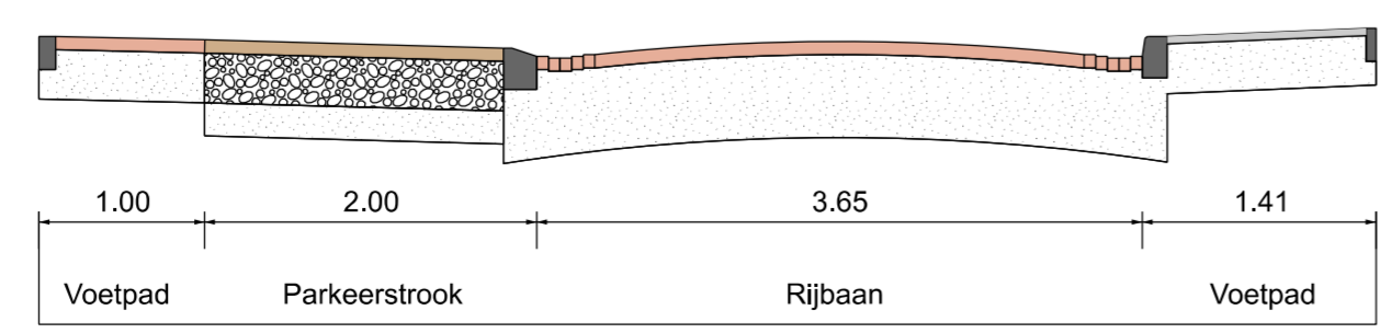
Dwarsprofiel A-A 1:50
